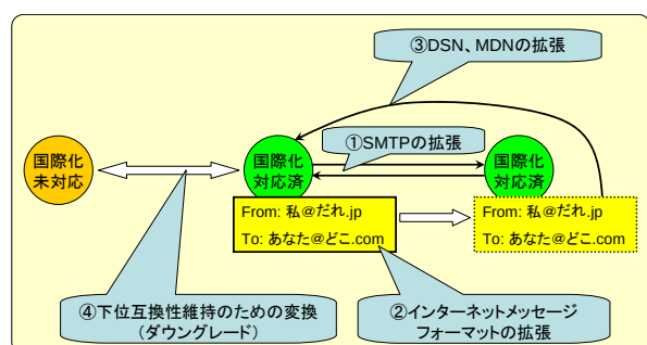
図1: EAI による電子メールアドレス国際化の概要
